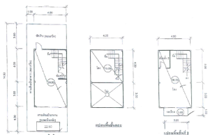
การผังผัง 1:100 (พื้นที่รวม 233.37 ตร.ม.)
