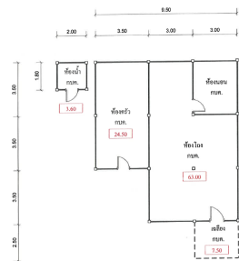
แปลนบ้านพักอาศัยที่ 30 หมู่ 4 ถนน 30
