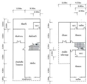
แปลนชั้นบน แปลนชั้นล่าง
