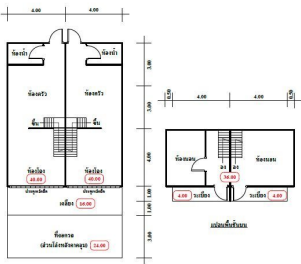
แปลนชั้นล่าง พื้นที่ใช้สอย 71.8 ตร.ม. (ใช้เป็นที่จอดรถ) จำนวน 0 ไร่ 0 งาน 71.8 ตารางวา
