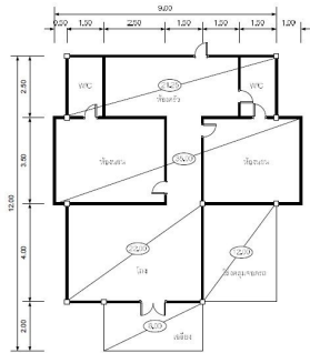
แบบแปลนอาคาร ชั้นบนสุด (รวมบันไดลอย) ชั้นล่างสุด (รวมบันได) ชั้นกลาง (รวมบันได)
