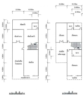
แบบแปลนสิ่งปลูกสร้าง 2 ชั้น เลขที่ 61
