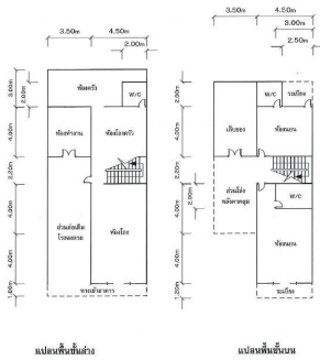
แบบแปลนสิ่งปลูกสร้าง 2 ชั้น เลขที่ 61
