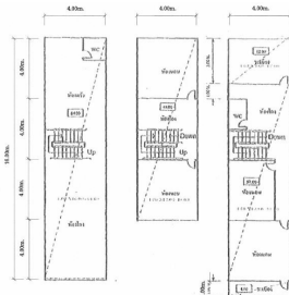
แบบแปลนอาคารชั้น 1 แบบแปลนอาคารชั้น 2 แบบแปลนอาคารชั้น 3
