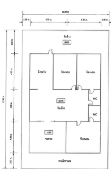
แบบแปลนบ้านเดี่ยวชั้นเดียว เลขที่ 219/105 จำนวน 1 หลัง
