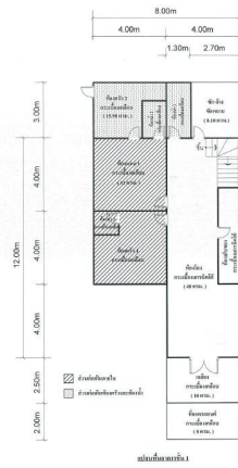
พื้นที่อาคารเดิม 2 ชั้น (ไม่ได้อยู่แล้ว)
